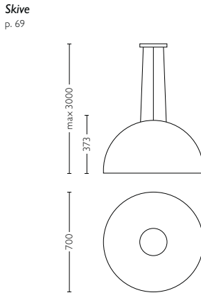
4038030LI class I, IP20, 230V H3000mm L700mm W700mm
