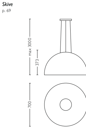
4038031LI class I, IP20, 230V H3000mm L700mm W700mm
